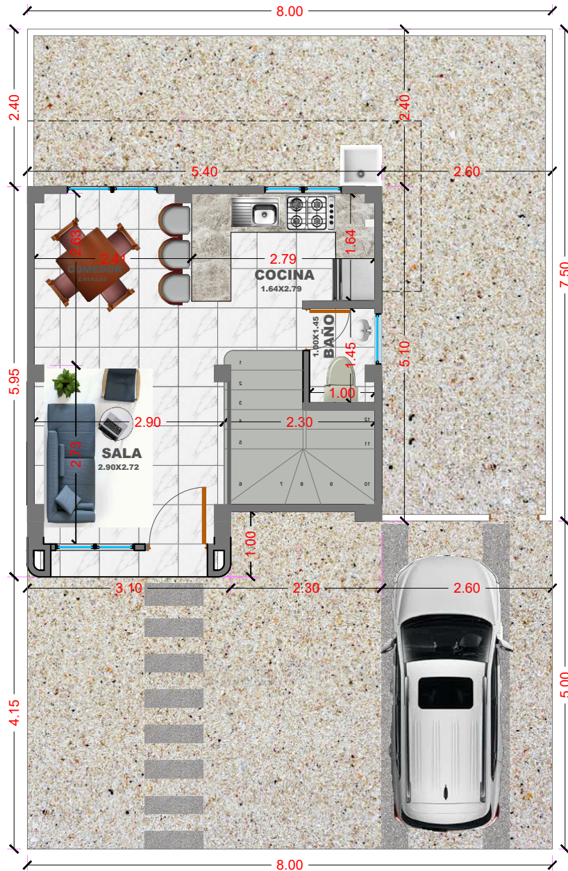
PLANTA ARQUITECTONICA VILLA MODELO SANTORINI PLANTA BAJA: 29.87m 2 TERRENO : 100.00m 2 VILLA : 65.62m 2
